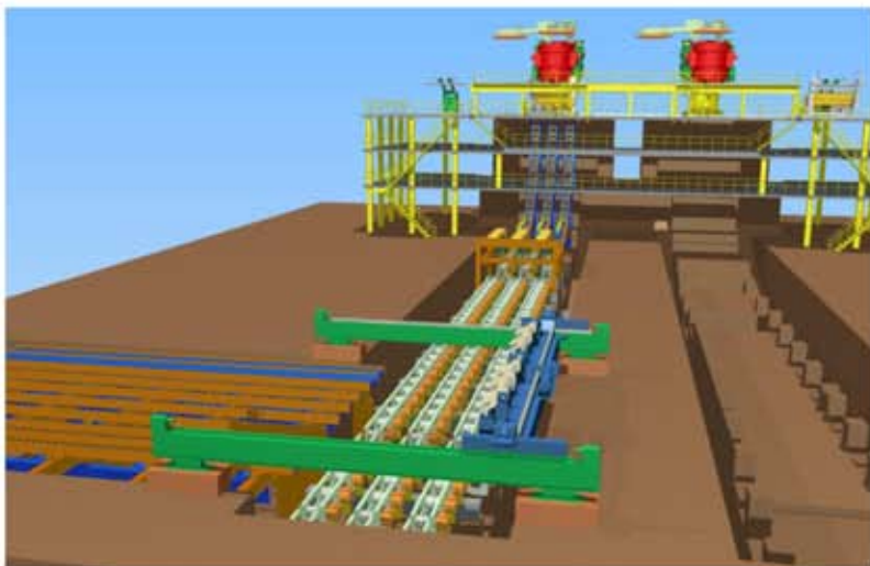
МНЛЗ
