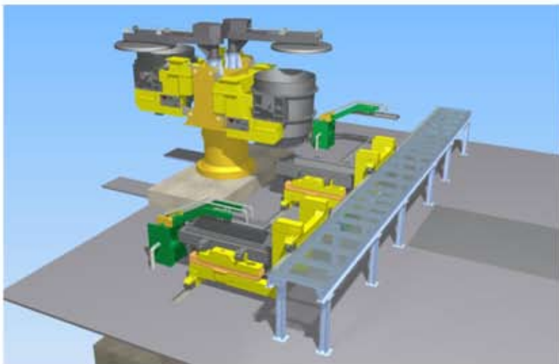
Поворотные стенды для установки и смены сталеразливочных ковшей в составе МНЛЗ
