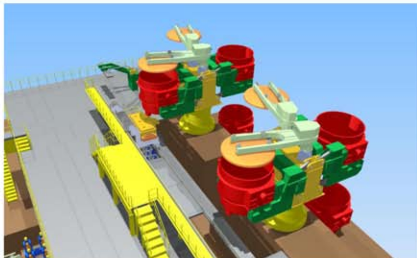
Поворотные стенды для установки и смены сталеразливочных ковшей в составе МНЛЗ
