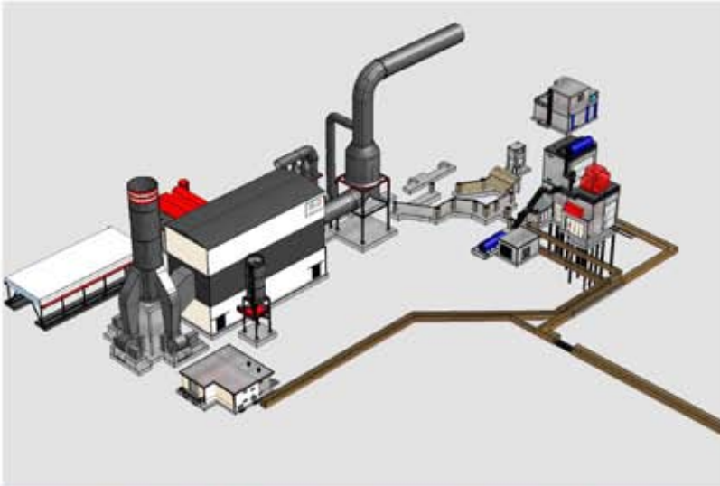
Интегрированный мини-металлургический завод
