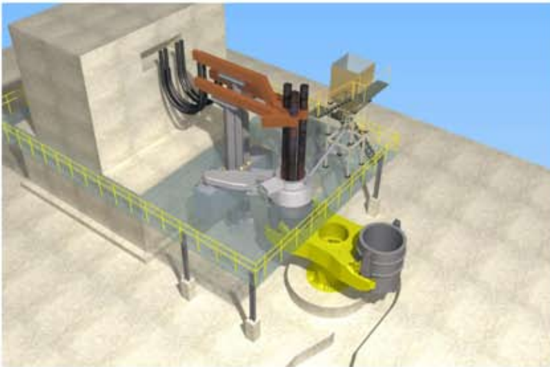
Агрегат "Печь-ковш"
